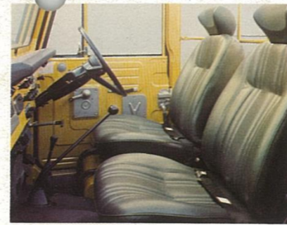
BJ40・43のフロントシート…ゆったりとしたヘッドレスト付セパレートシート。2点式シートベルトも装備。
