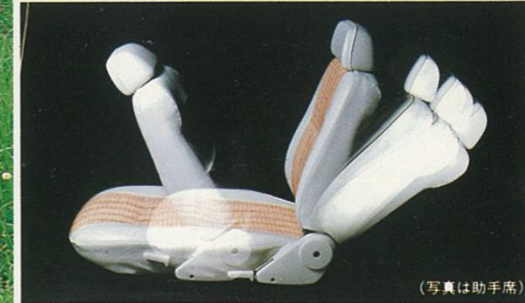
リクライニングシート。どなたでも最適なドライビングポジションが選べるリクライニングシート。座り心地も乗り心地も一段と向上しています。(BJ41V、44V)
