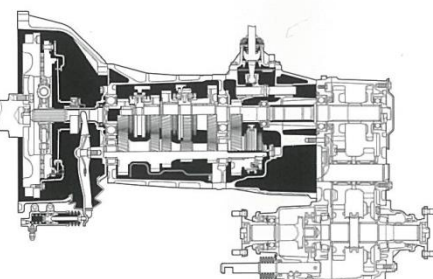
5速マニュアルトランスミッション
