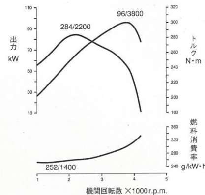
LASRE 1HZ DIESEL 性能曲線図
