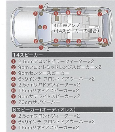
スピーカーレイアウト
